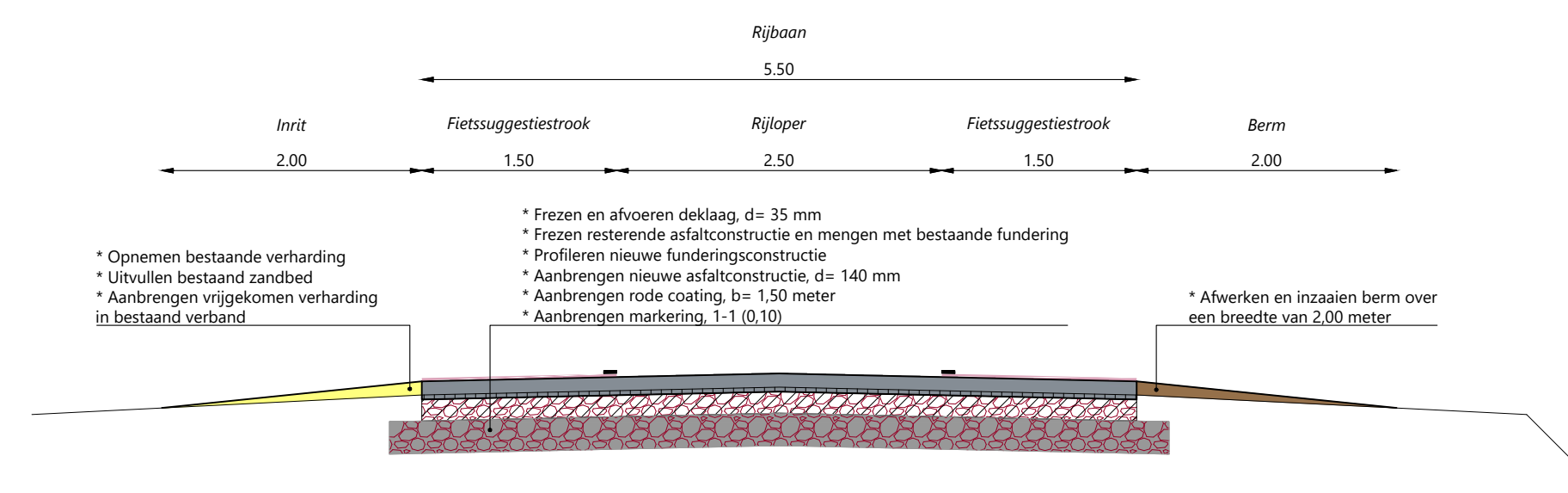
PRINCIPE PROFIEL MAATREGEL BURGEMEESTER STROINKSTRAAT Schaal 1:50
