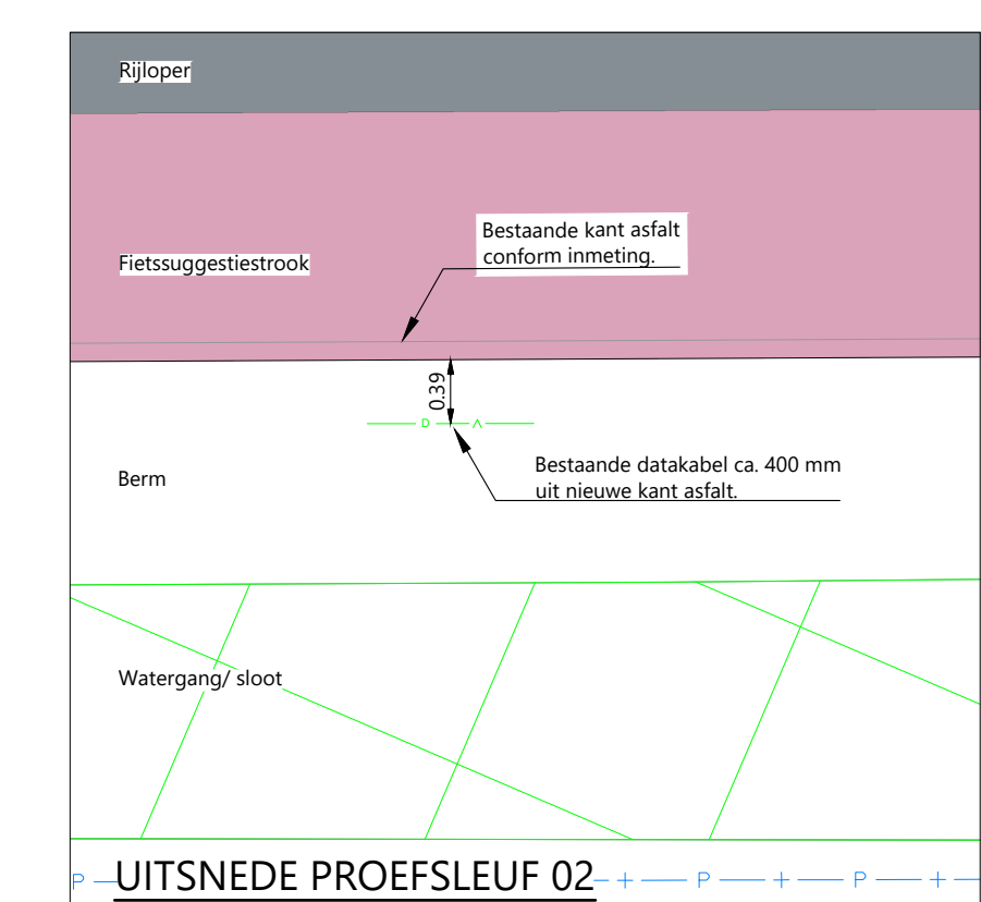
UITSNEDE PROEFSLEUF 02 Schaal 1:50
