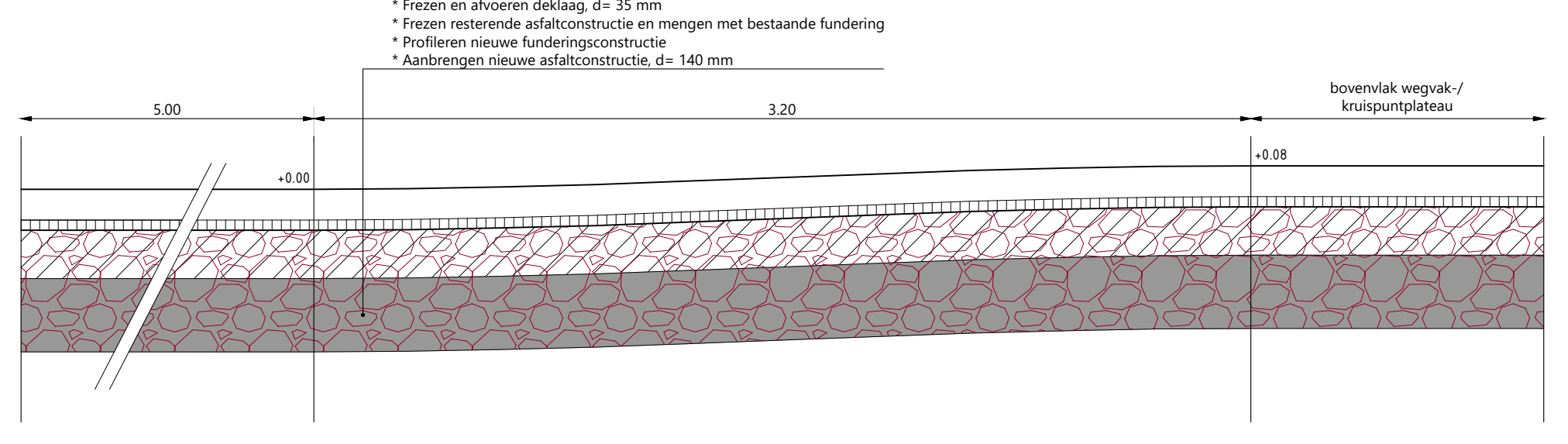
PRINCIPE LENGTEPROFIEL RECONSTRUCTIE BESTAANDE DREMPEL Schaal 1:50
