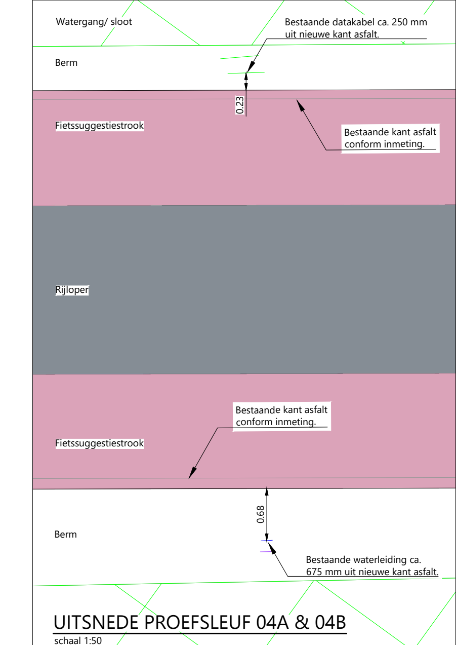
UITSNEDE PROEFSLEUF 04A & 04B Schaal 1:50
