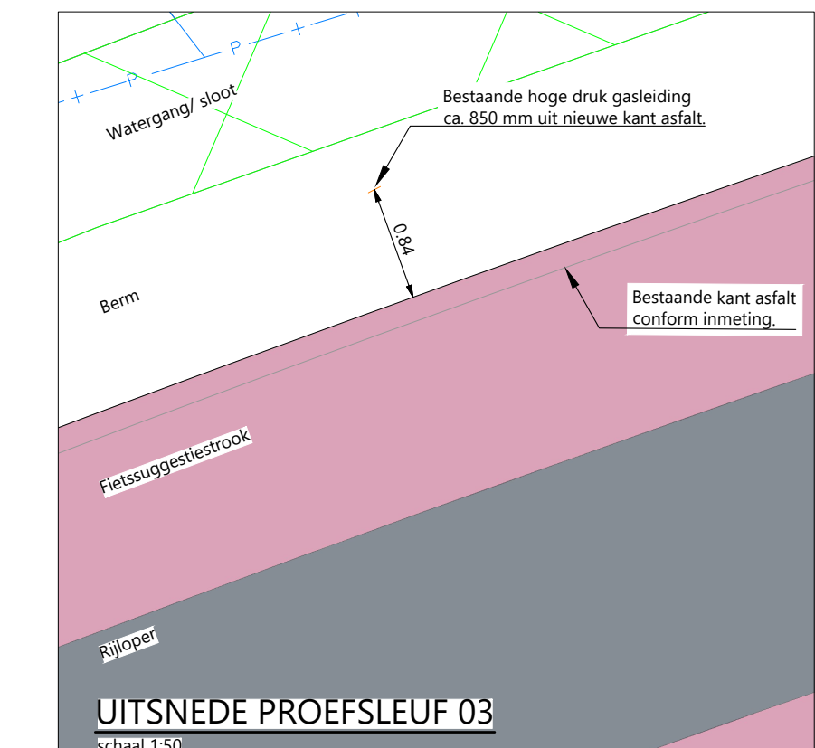
UITSNEDE PROEFSLEUF 03 Schaal 1:50
