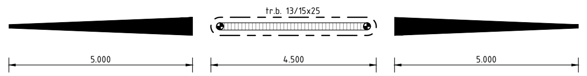
Detail: wegversmalling Schaal 1:100
